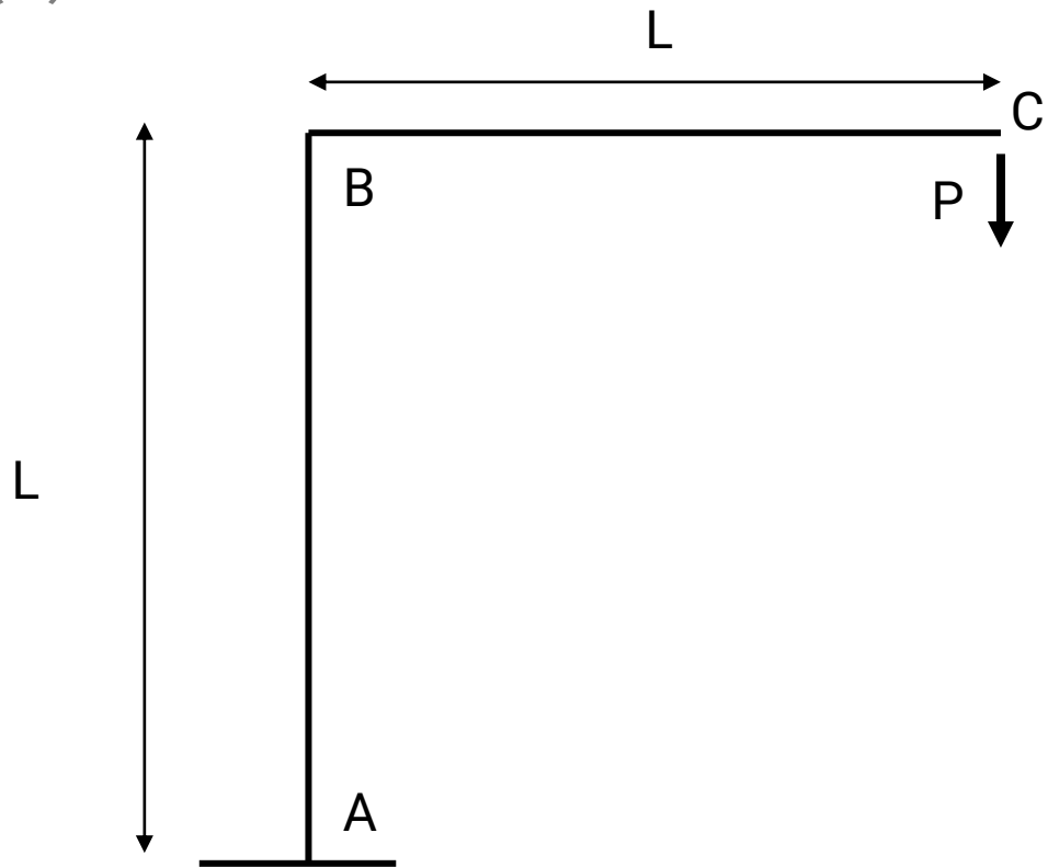
片持梁型
