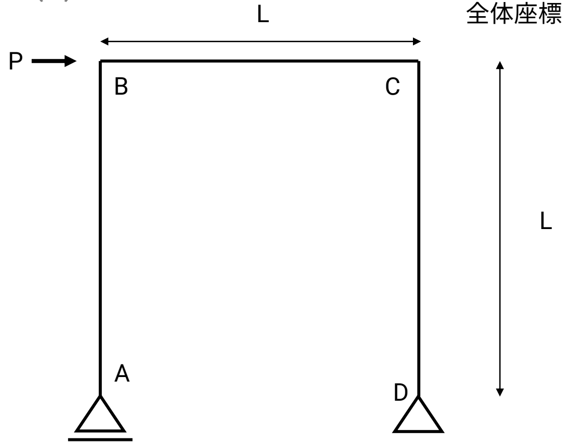
単純支持型
