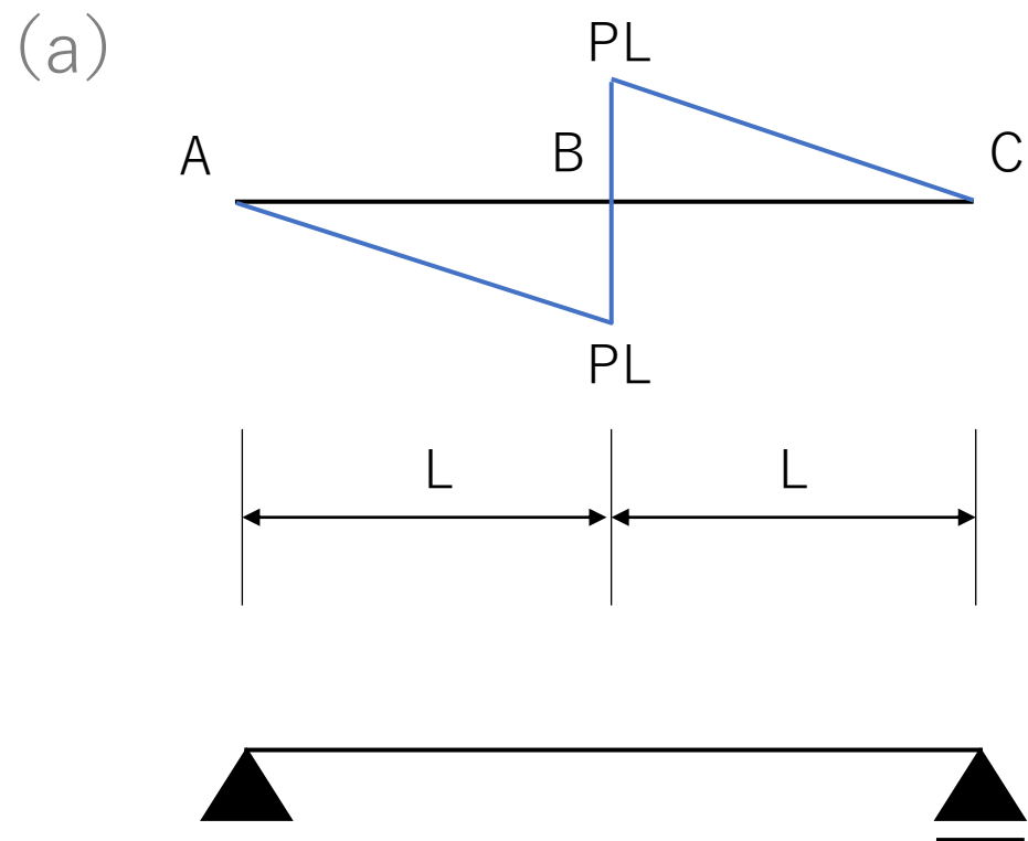
全体釣合図
