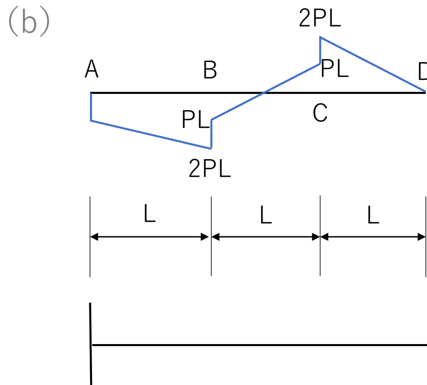
全体釣合図
